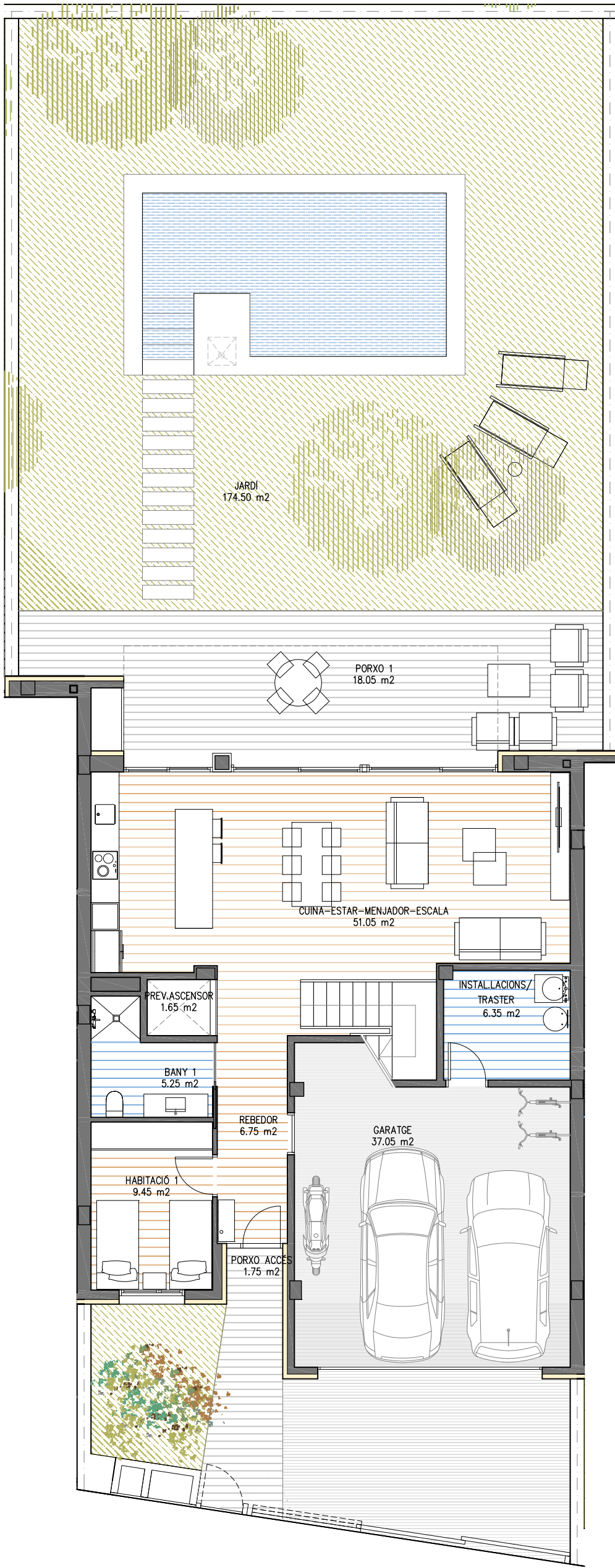
PL. BAIXA
