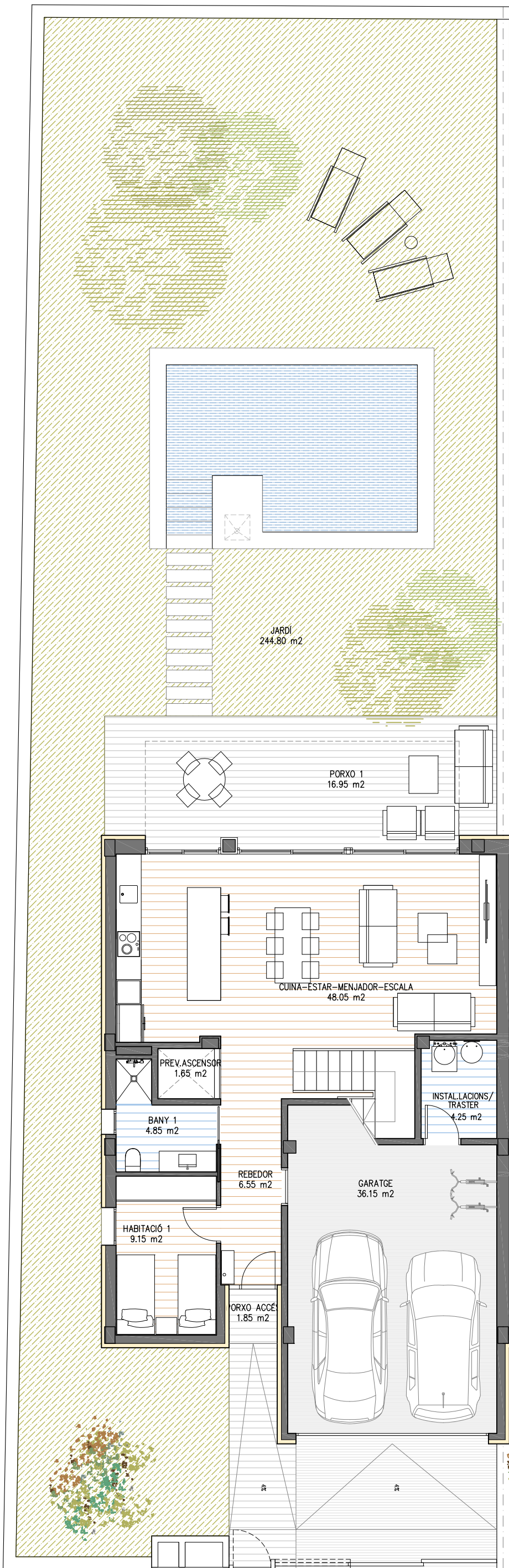
PL. BAIXA
